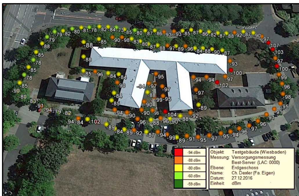
Abbildung 18: Umfeldmessung LMR Master m. GPS (Google Earth)
