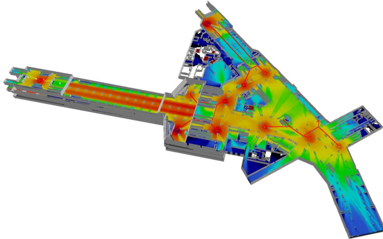
Abbildung 13: Inhouse-Versorgungssimulation (Beispiel)
